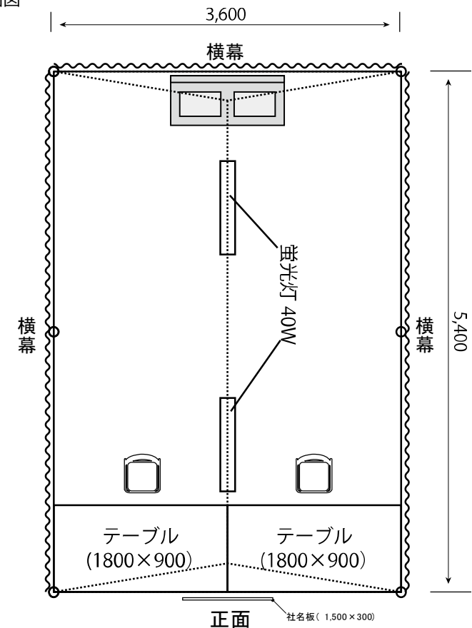
平面図
